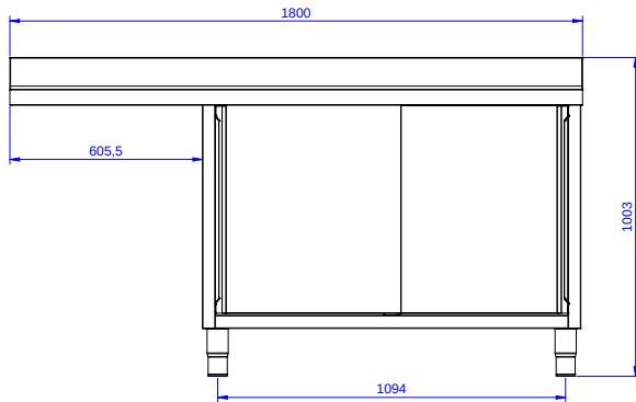
Zij aanzicht
